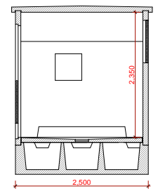
Corte A-B (lay-out 2Gb)
