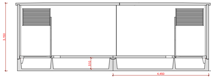
Corte C-D (lay-out 2Ga)
