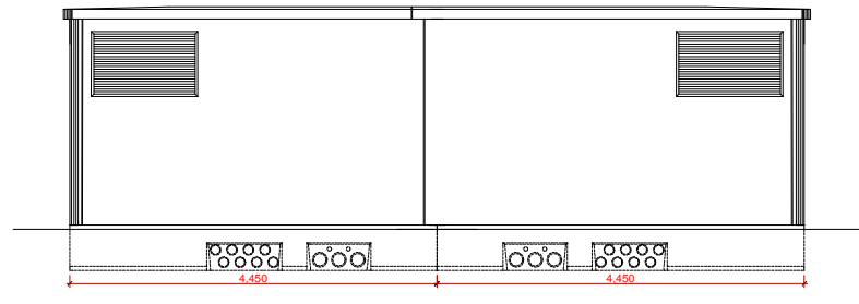
Alçado Posterior
