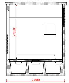
Corte A-B (lay-out 2Ga)
